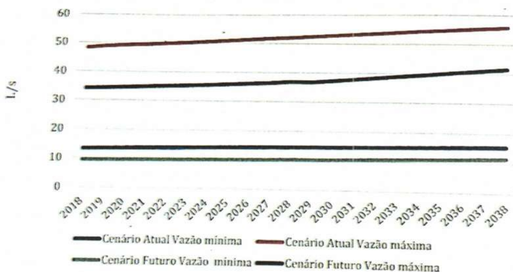
Figura 16 – Vazões estimadas – cenário atual e futuro
