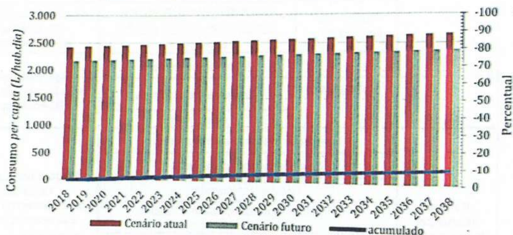
Figura 8 – Projeções do consumo nos cenários atual e futuro
